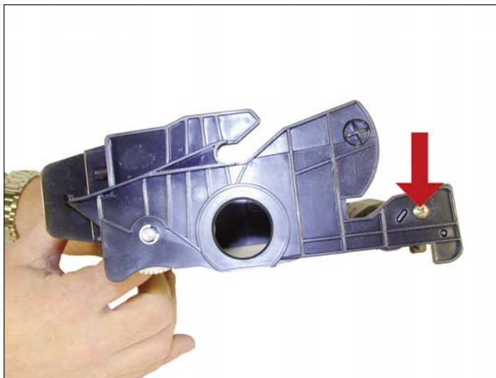
1. Remueva los dos tornillos de ambos lados de la manija/candado del cartucho.
