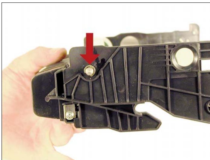
3. Remueva el anillo-E del lado de los engranajes pequeños del eje del cilindro.
